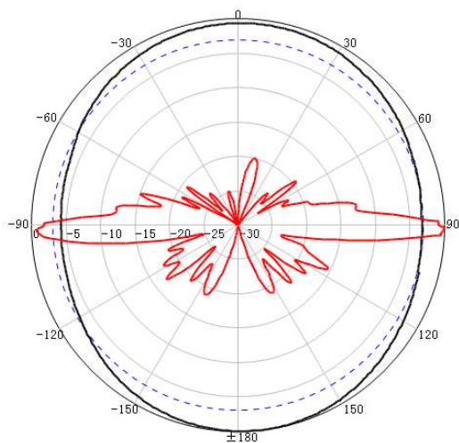
H-Pol @ 2450MHz
